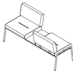
DOUBLE BENCH AVEC TABLETTE CENTRALE | WITH MIDDLE TRAY (FACE-TO-FACE) 1.675 x 704 x 783 mm
