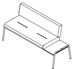
DOUBLE BENCH AVEC TABLETTE LATÉRALE | WITH SIDE TRAY 1.675 x 655 x 783 mm
