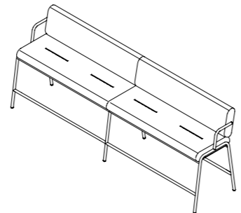
2 X DOUBLE BENCH AVEC PIED DE CONNEXION | WITH CONNECTING LEG 2.650 x 605 x 998 mm
